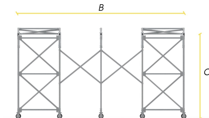
PROSPETTO LATERALE
