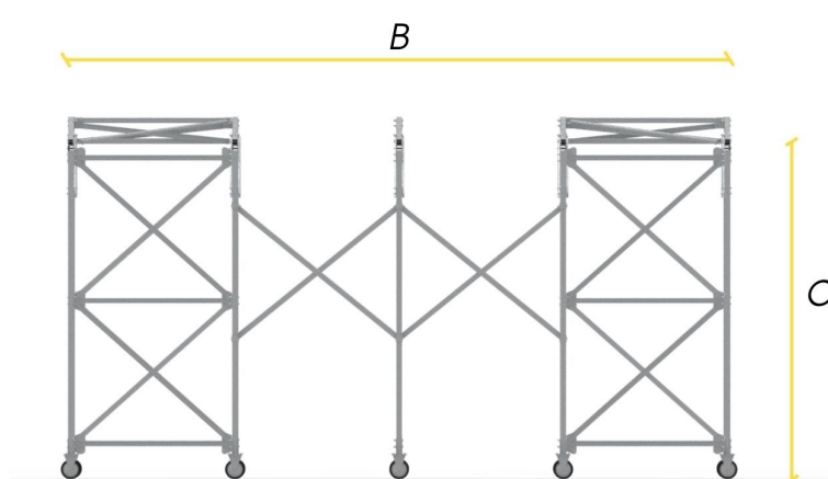
PROSPETTO LATERALE
